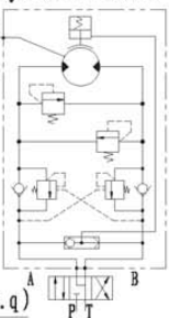
液压原理图 Hydraulic chart
