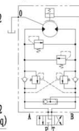
液压原理图 Hydraulic chart
