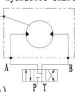
液压原理图 Hydraulic chart
