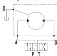
液压原理图 Hydraulic chart
