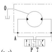
液压原理图 Hydraulic chart
