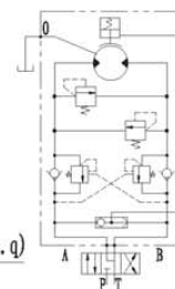
液压原理图 Hydraulic chart
